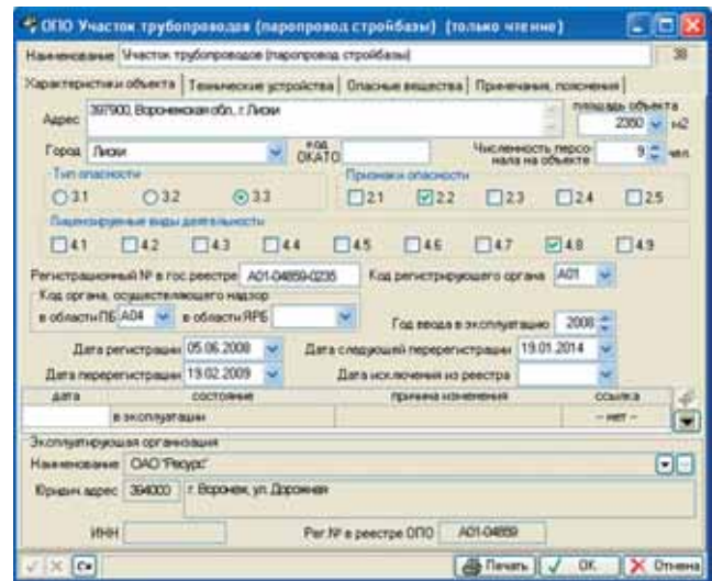
▲ Рис. 1. Карточка опасного производственного объекта
