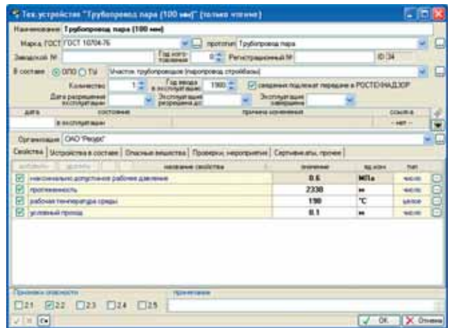
▲ Рис. 2. Карточка технического устройства
